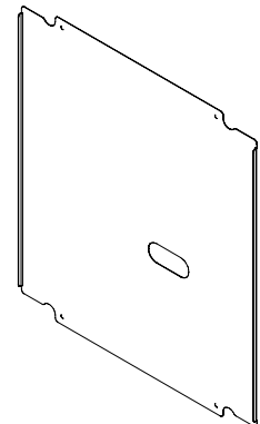
Bottom Panel 05700-003-32-92
